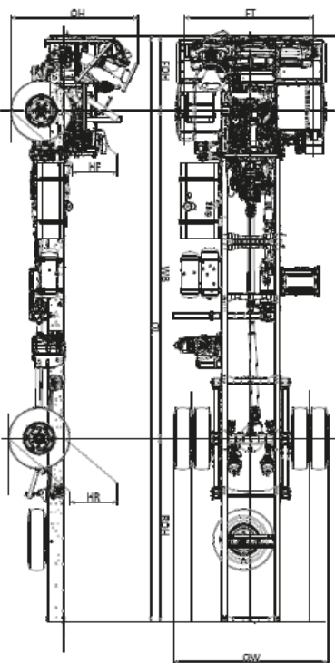
Dimensiones (mm)
